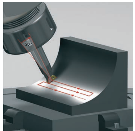
Bearbeitung mit Sturzwinkel
