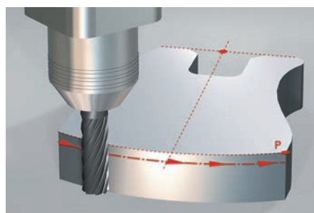
RND Ecken-Runden: Kreisbahn mit beidseitig stetigem (tangentialem) Anschluss, festgelegt über Radius und Eckpunkt
